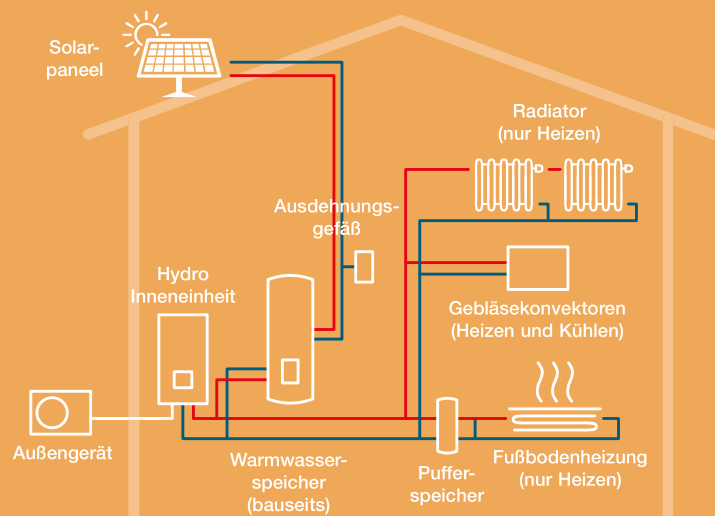
2 Zonen mit Solar- und Kühlfunktion in einem Neubau
